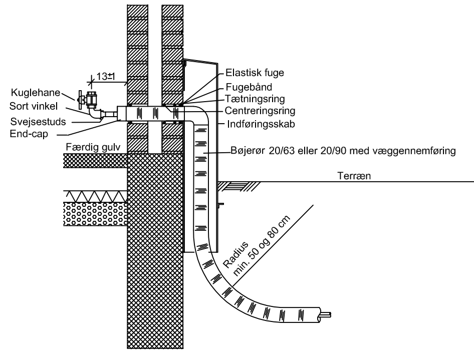
Stikindføring C. med bøjerør 20/63 og 20/90
