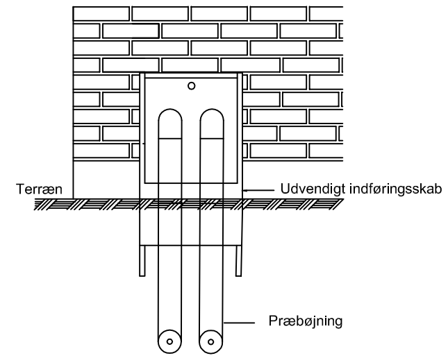
Opstalt af indføringsskab.
