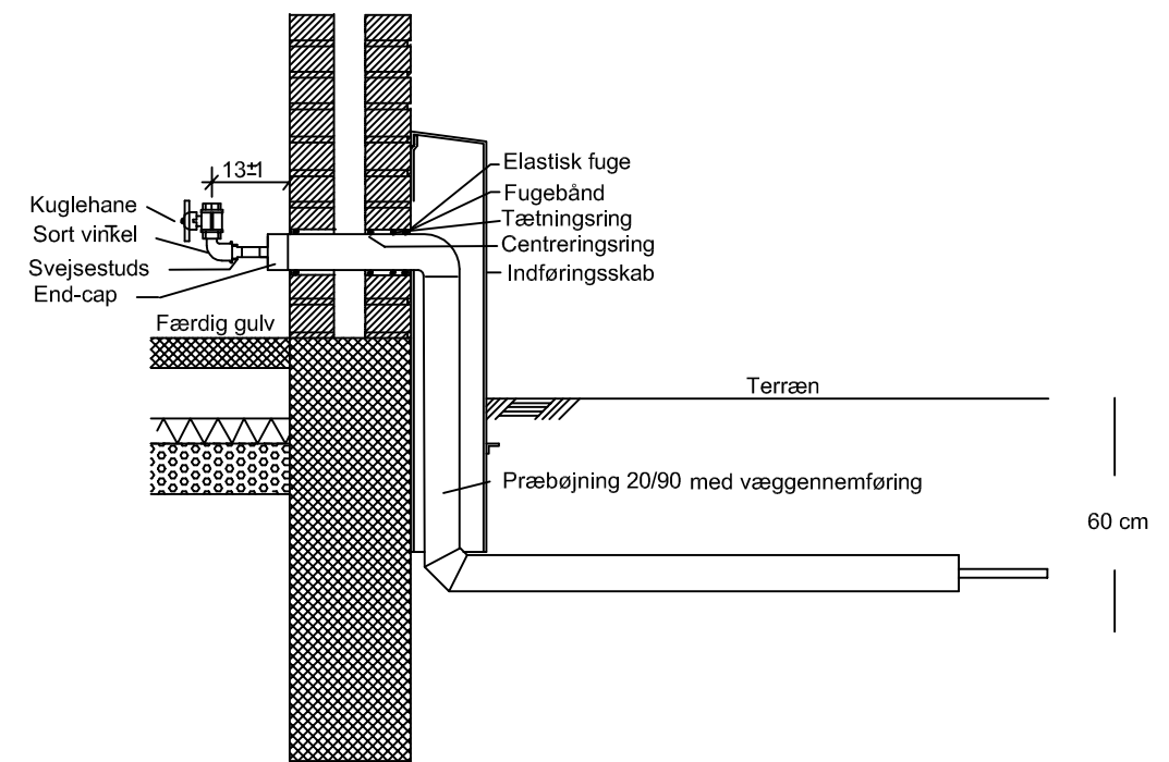
Stikindføring C. med præbøjning 20/90 med væggennemføring
