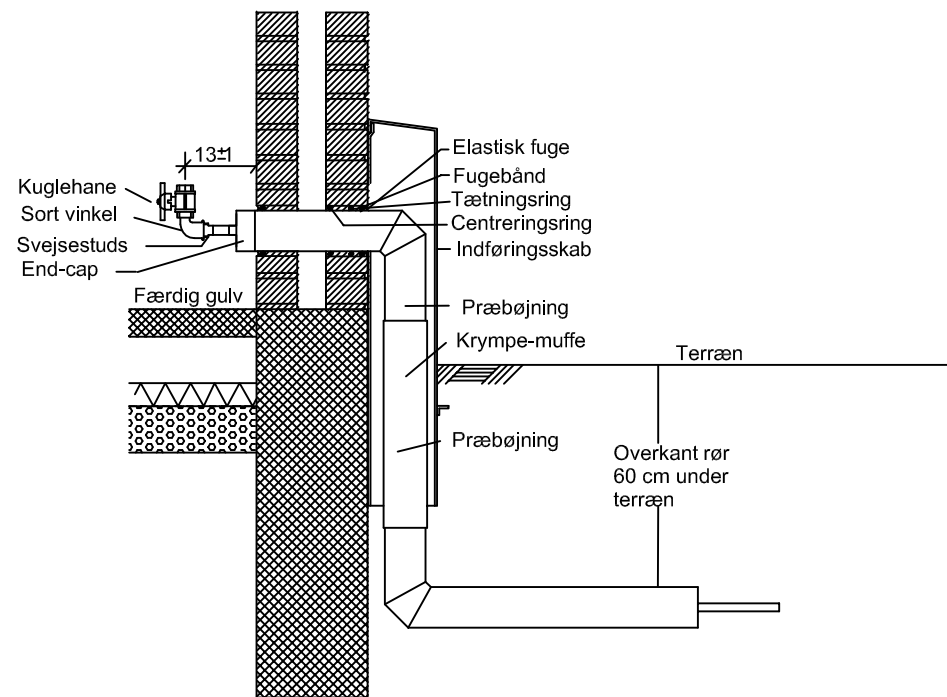
Stikindføring C1. med præbøjning NW20 til NW32
