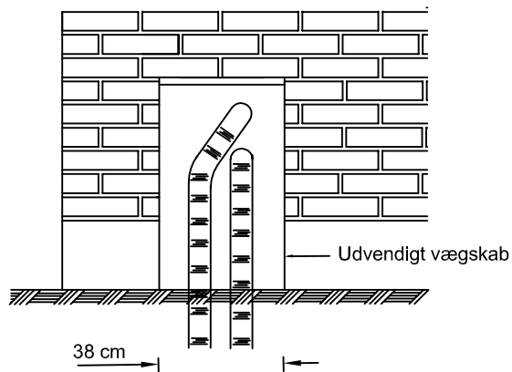
Opstalt af indføringsskab
