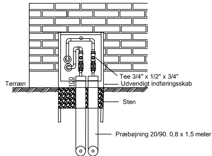
Opstalt af indføringsskab med indføring i gulvpanel.
