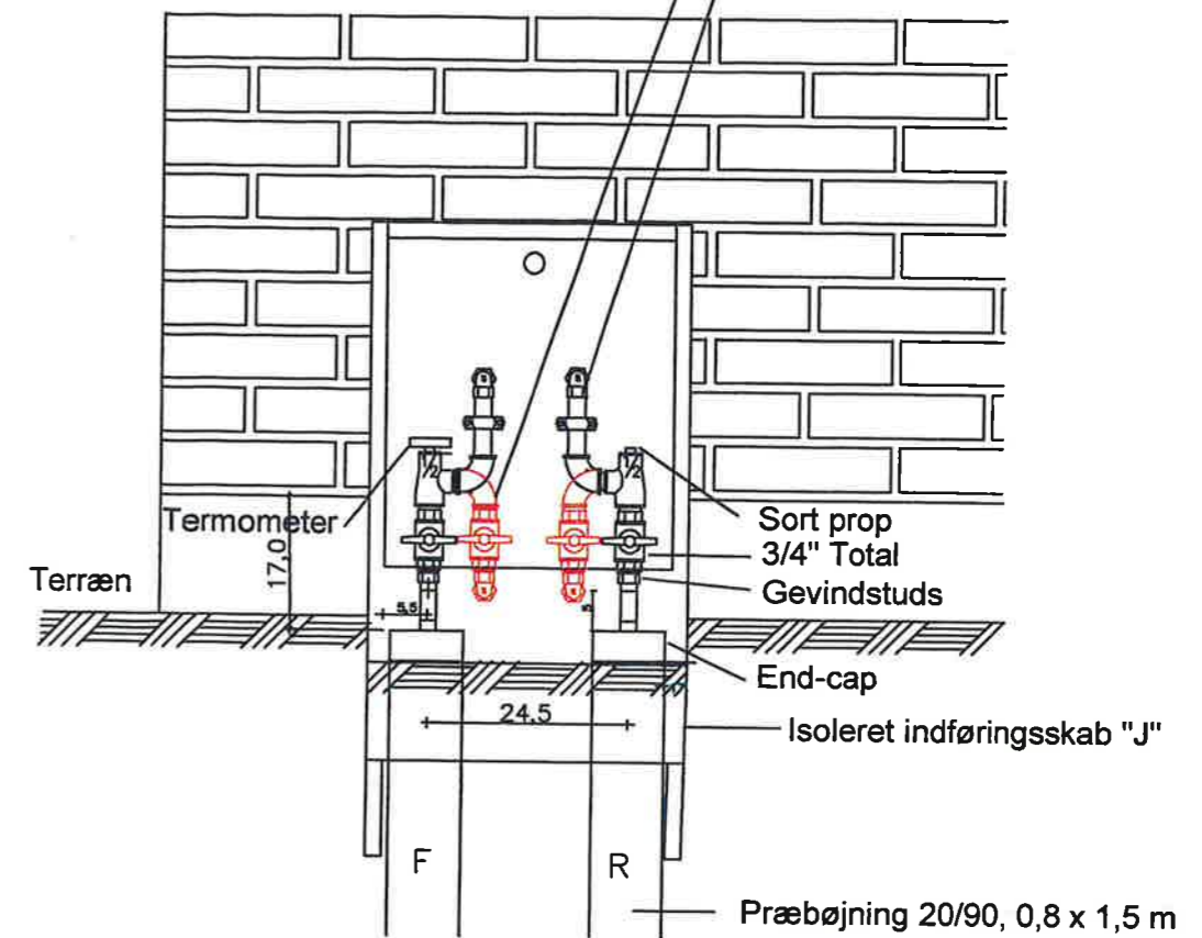
Lodret snit
