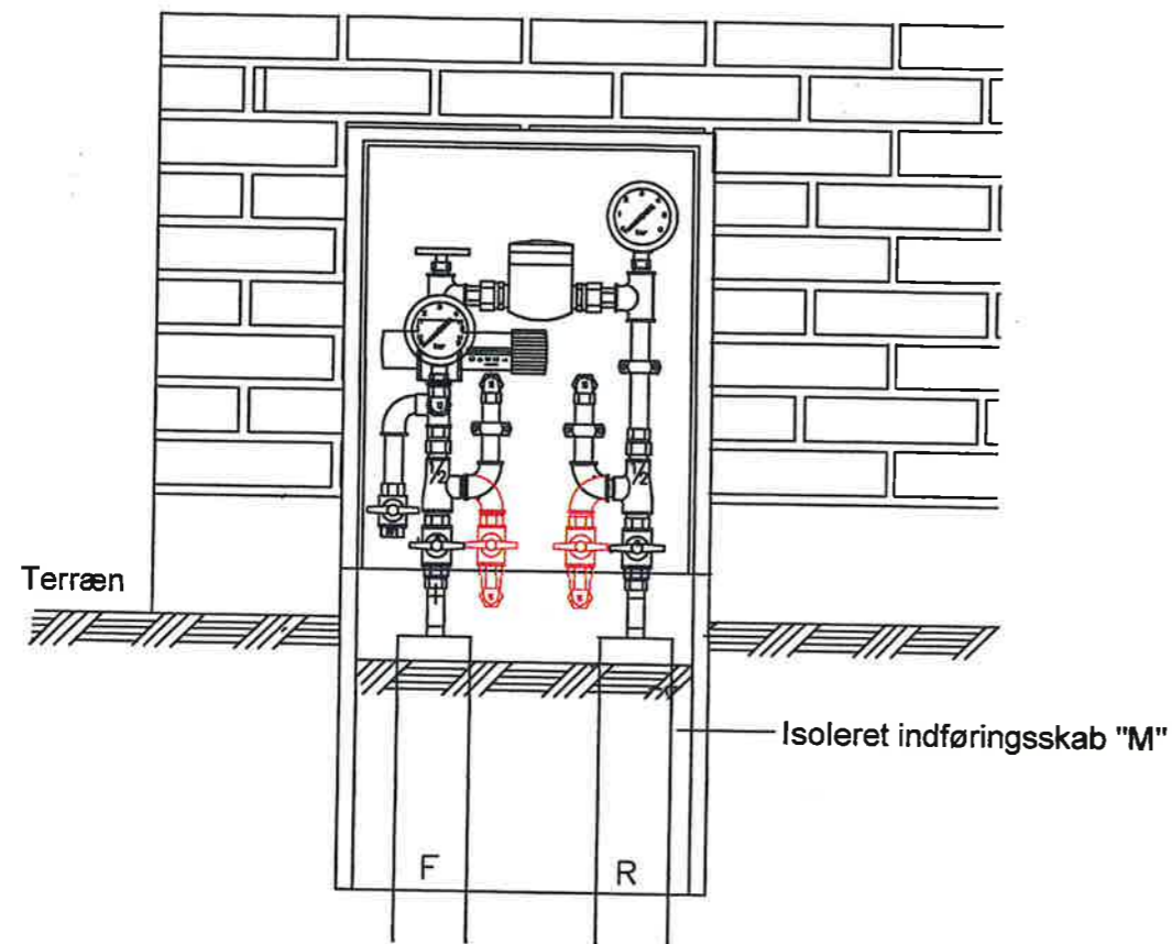
Lodret snit
