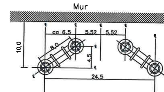
Vandret snit i stikindføring 1 : 5.
